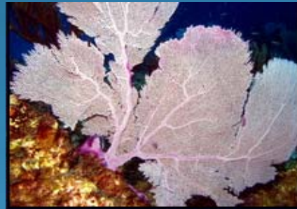
Common Sea Fan
